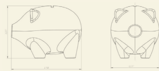
Создаем габаритный чертеж копилки
